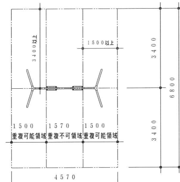
安全領域図 S = 1 / 100
