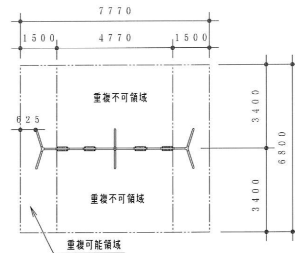
安全領域図 S = 1 / 150
