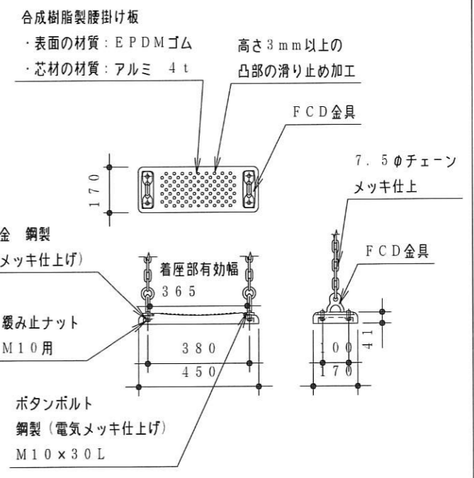
座板詳細 S = 1 / 20
